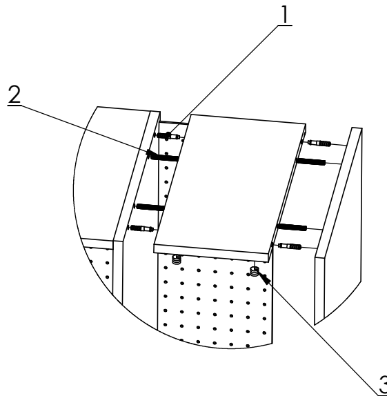
DETALLE C ESCALA 1 : 10
